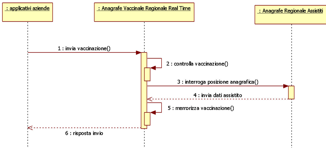
Figura 4 – sequence diagram FB - trasmissione vaccinazione
